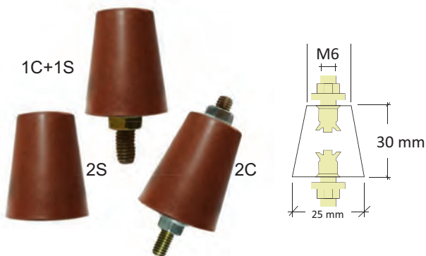
MİNİ BOY KONİK İZOLATÖR MINI SIZE CONICAL INSULATOR
