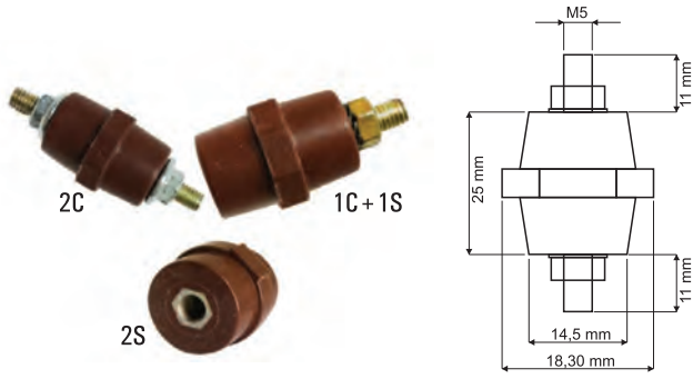
M5 MİNİ İZOLATÖR 25mm M5 MINI INSULATOR 25mm
